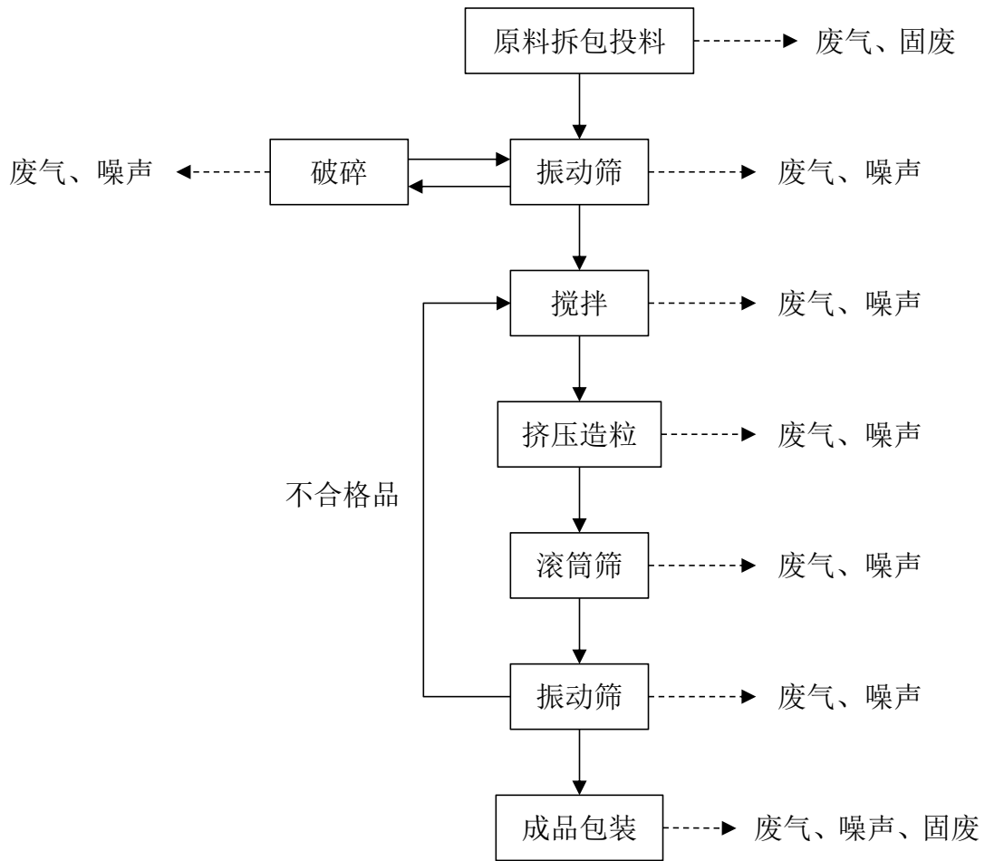
图 2-2 复混肥料生产工艺流程及产排污环节示意图
