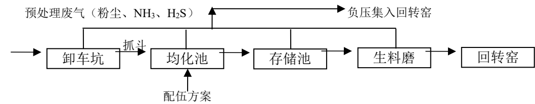
图 2.10-1 固体废物预处理工艺流程图
