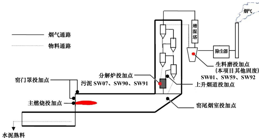
图 2.10-3 本项目固废投加点示意图
