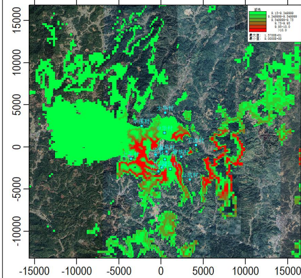
正常排放 NO 2 叠加年平均浓度分布图(μg/m 3 )
