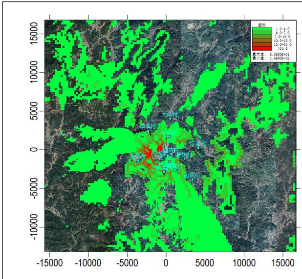
正常排放 NO 2 贡献日均浓度分布图(μg/m 3 )
