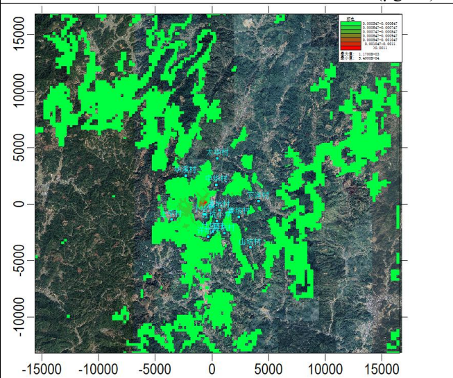
正常排放氟化物叠加日平均浓度分布图( \mu\text{g}/\text{m}^3 )
