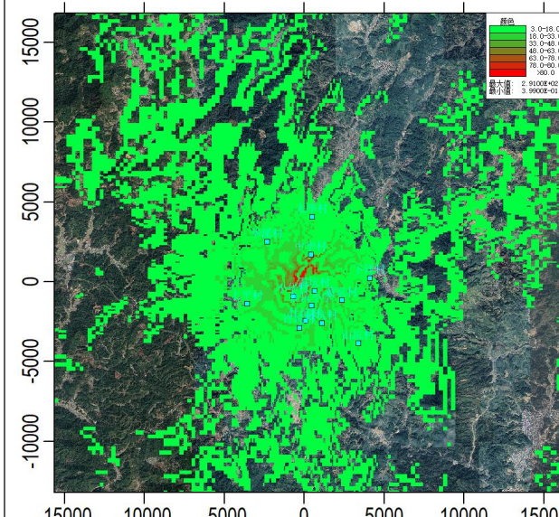
正常排放 PM 10 贡献小时浓度分布图(μg/m 3 )
